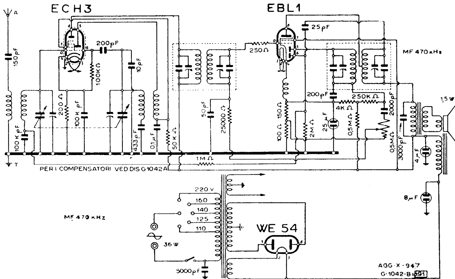
F.I.M.I. - MOD. PHONOLA « 301/2 »
